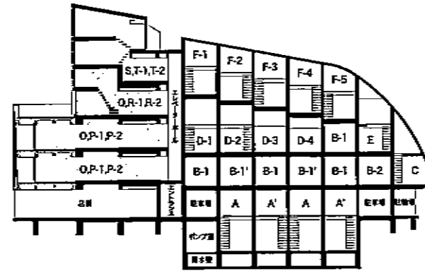
断面図
