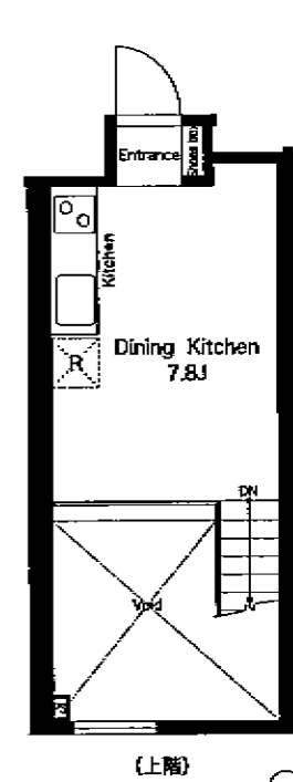
Atype 1DK | 46.80㎡(14.15坪)
