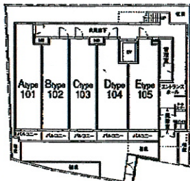
1階平面図
