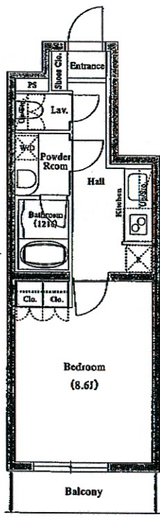
2,3階平面図
