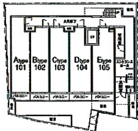
1階平面図
