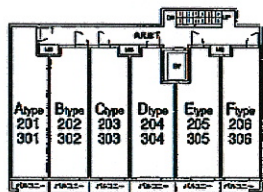
2,3階平面図
