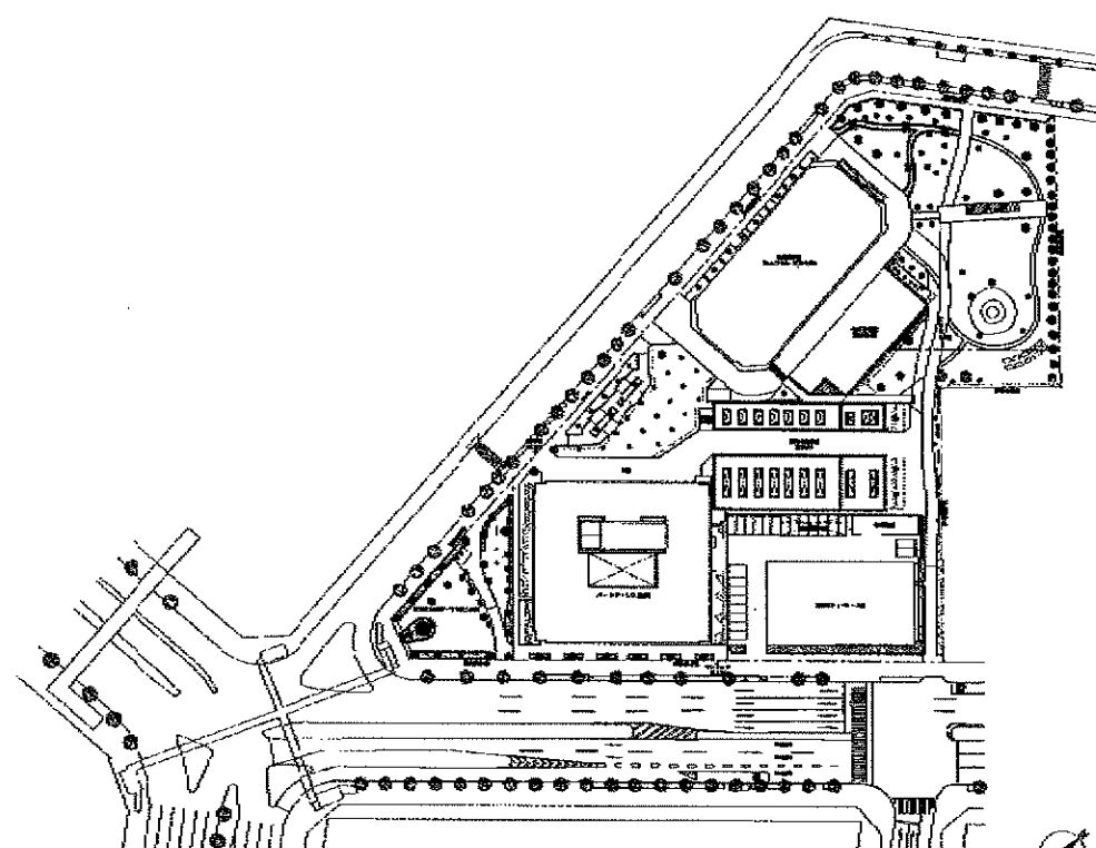
《敷地配置図》
