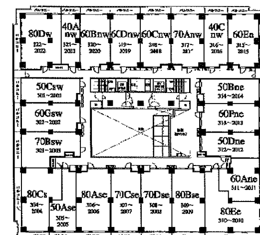
《3-20F 平面図》
