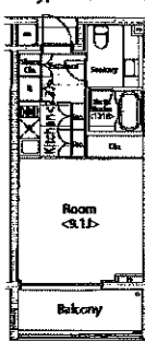
■ K1-type 1K / 29.60㎡(8.95坪)
